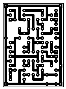
【基板転写用】 (実寸・左右反転済)
